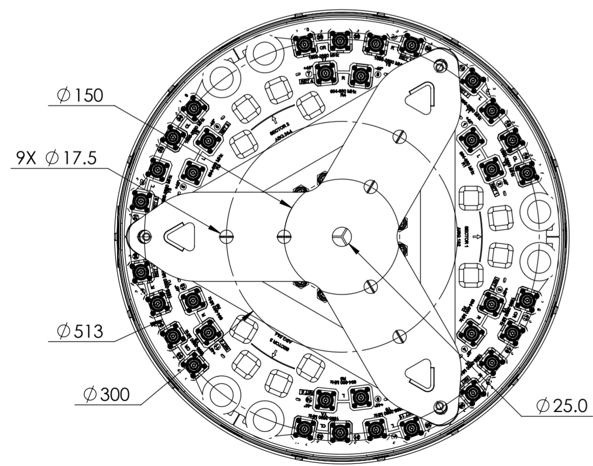
VIEW A-A
