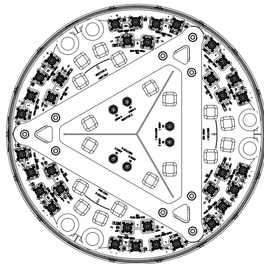
VIEW A-A BOT BKT NOT SHOWN
